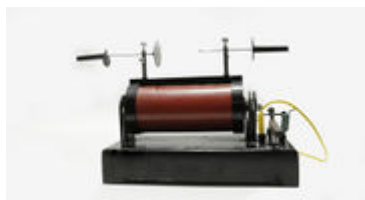
Ruhmkorffův transformátor
