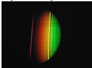
Spektrum vodík
