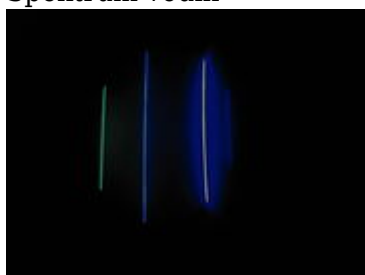
Spektrum helium
