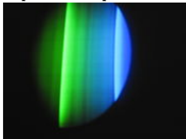
Spektrum CO 2
