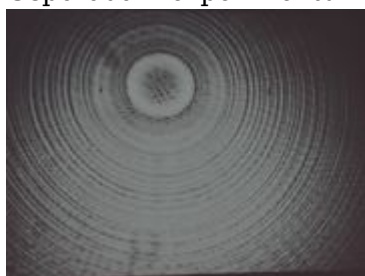
Interferenční obrazec
